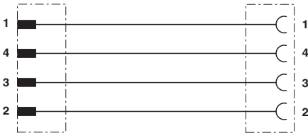
M12针式和M12孔式的触点分配
