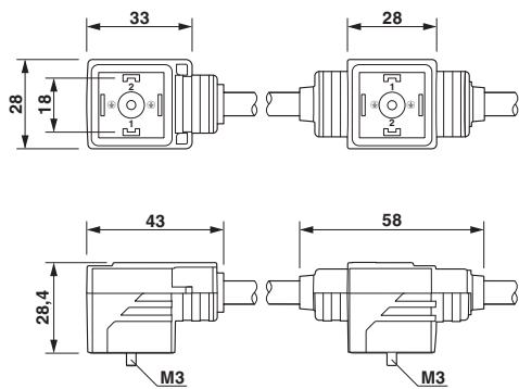
尺寸图
