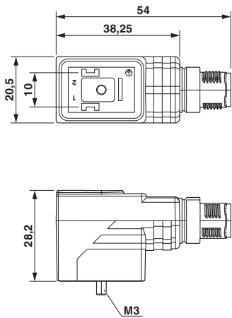
尺寸图
