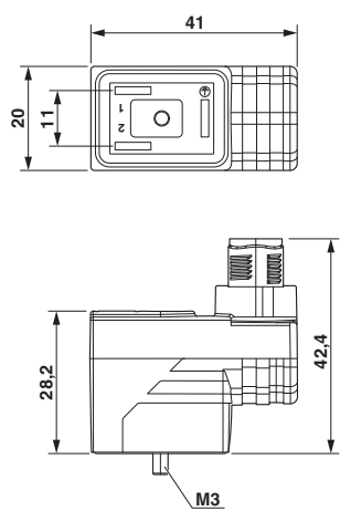
尺寸图
