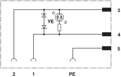
电路图
