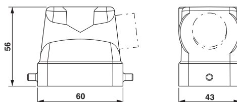
尺寸图
