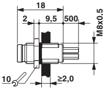
尺寸图
