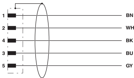
电路图
