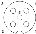
M12孔式连接器引脚分配，5芯，A编码，插座侧视图
