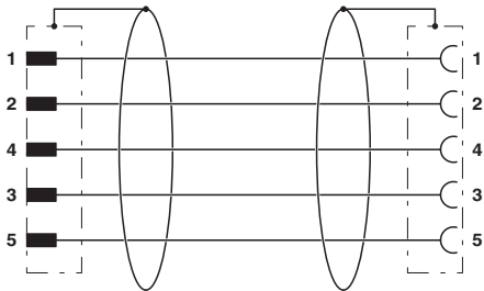
电路图
