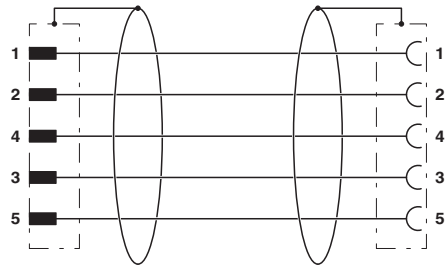
电路图
