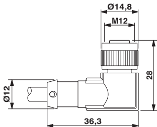
尺寸图
