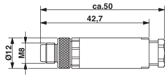
尺寸图
