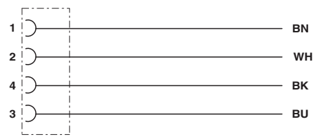
电路图
