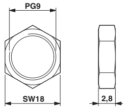
尺寸图
