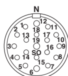
M23孔式引脚分配，19芯，插座侧视图
