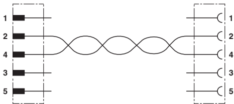
电路图
