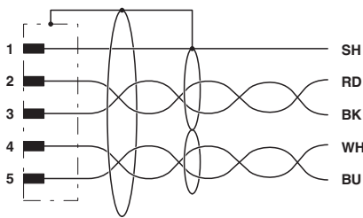
电路图
