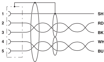
电路图
