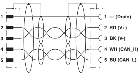
M12针式和M12孔式连接器的触点分配
