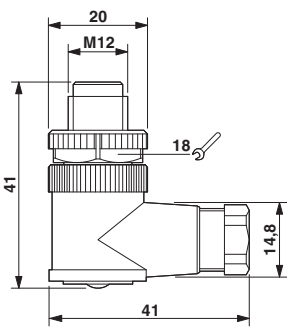
尺寸图
