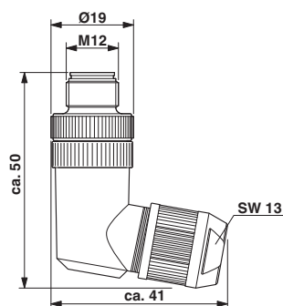
尺寸图
