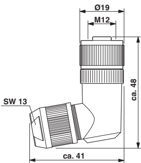
尺寸图
