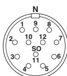
M23孔式引脚分配，12芯，插座侧视图
