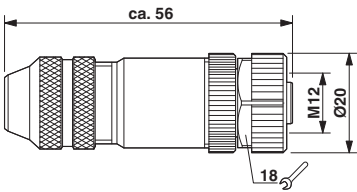
尺寸图
