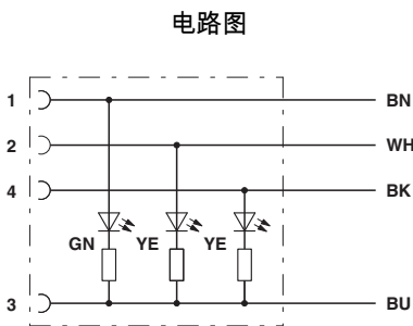
带有2个LED的M12孔式连接器的触点分配，
