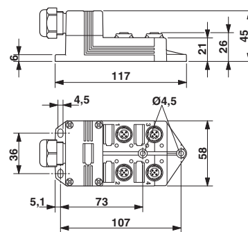
尺寸图
