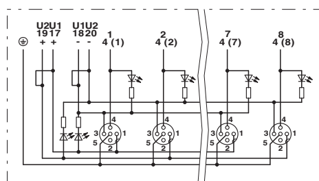
电路图
