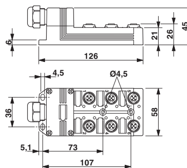
尺寸图
