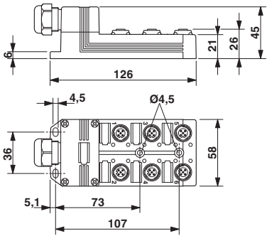
尺寸图
