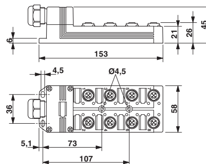
尺寸图
