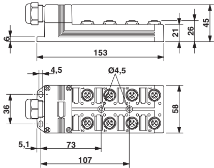
尺寸图
