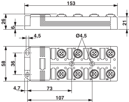
尺寸图
