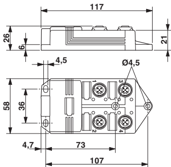
尺寸图
