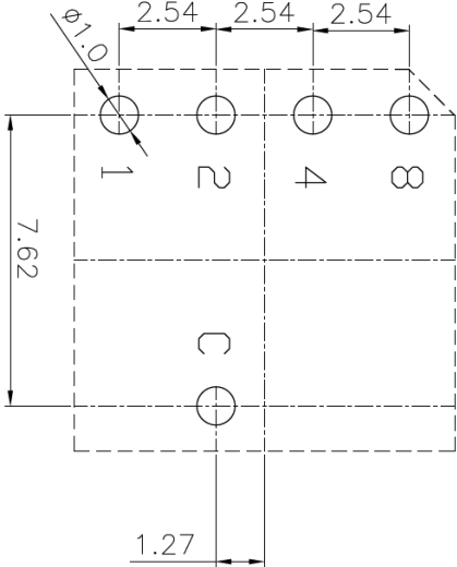
P.C.B. DIMENSION
