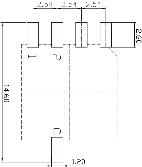
P.C.B DIMENSION
