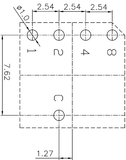
P.C.B DIMENSION
