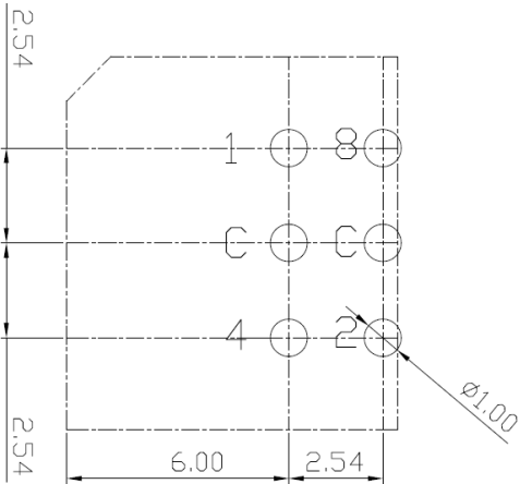
P.C.B. DIMENSION
