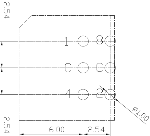
P.C.B. DIMENSION
