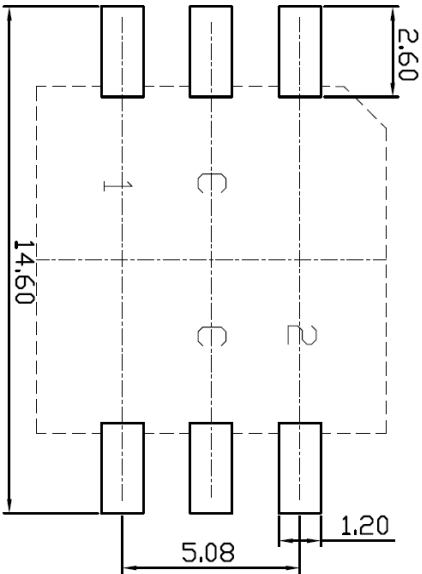
P.C.B DIMENSION
