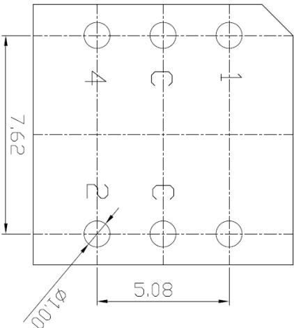
P.C.B. DIMENSION
