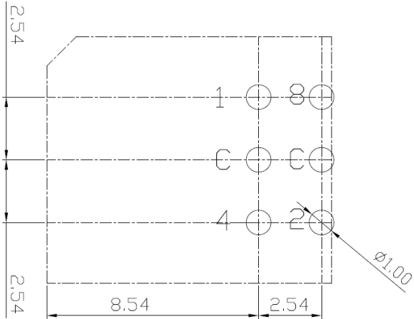
P.C.B. DIMENSION
