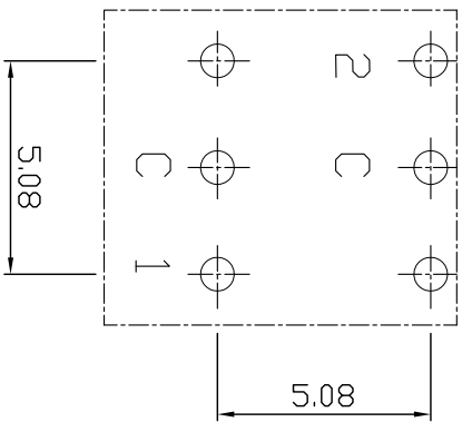
P.C.B DIMENSION
