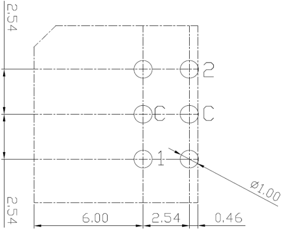
P.C.B DIMENSION
