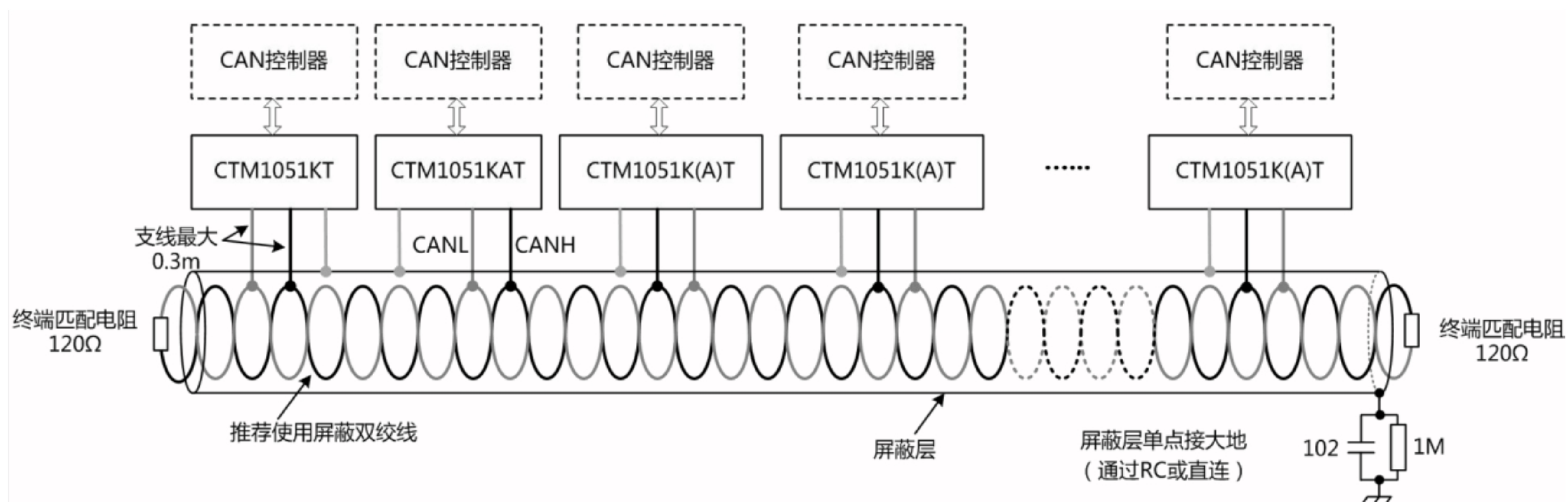
图3.单个CAN-Bus典型网络连接示意图
