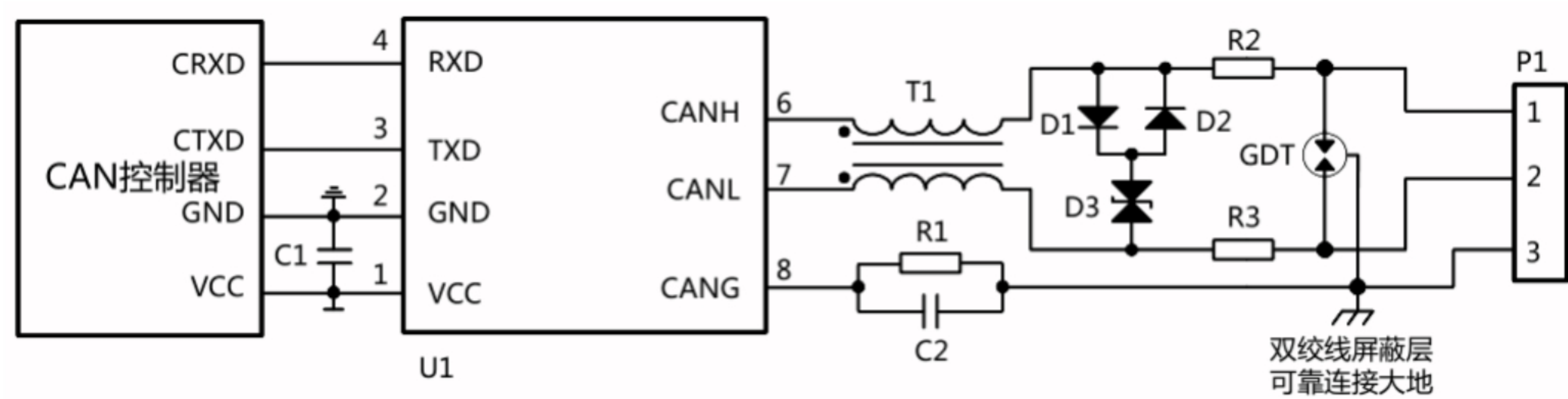
图4. EMC推荐电路
