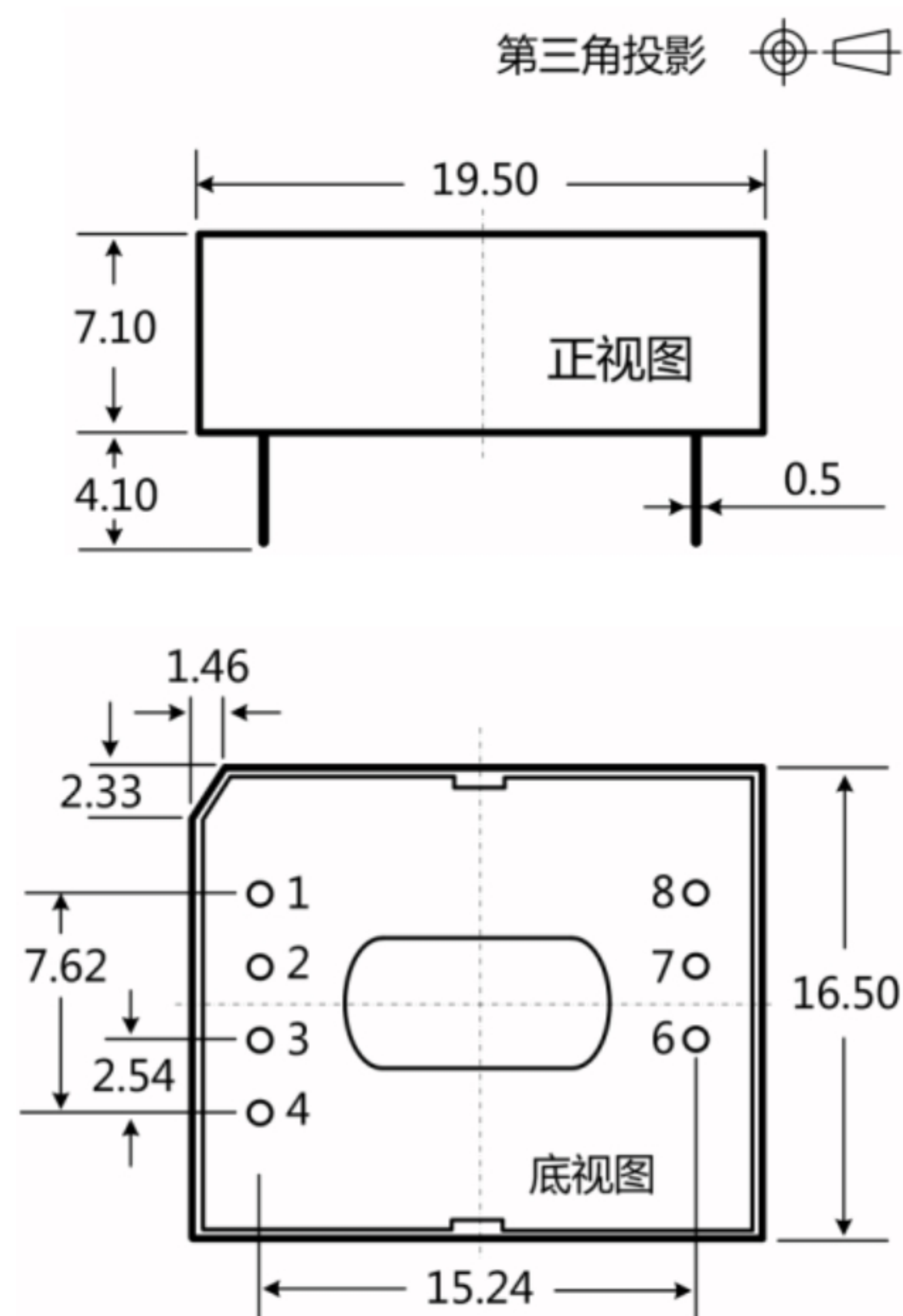
外观尺寸图
