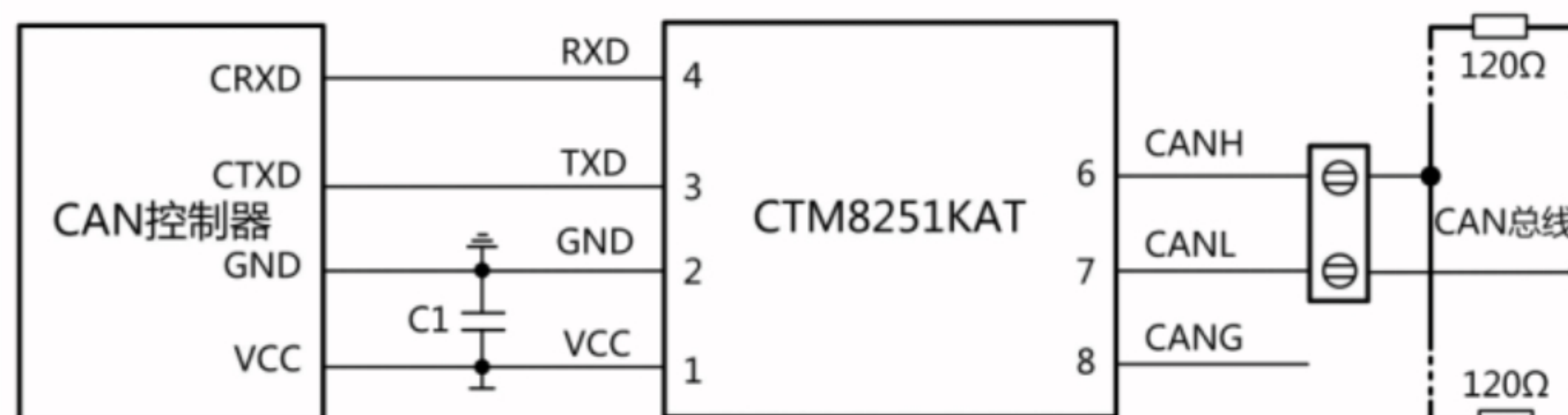
图 2. CAN 控制器 3.3V 供电应用电路
