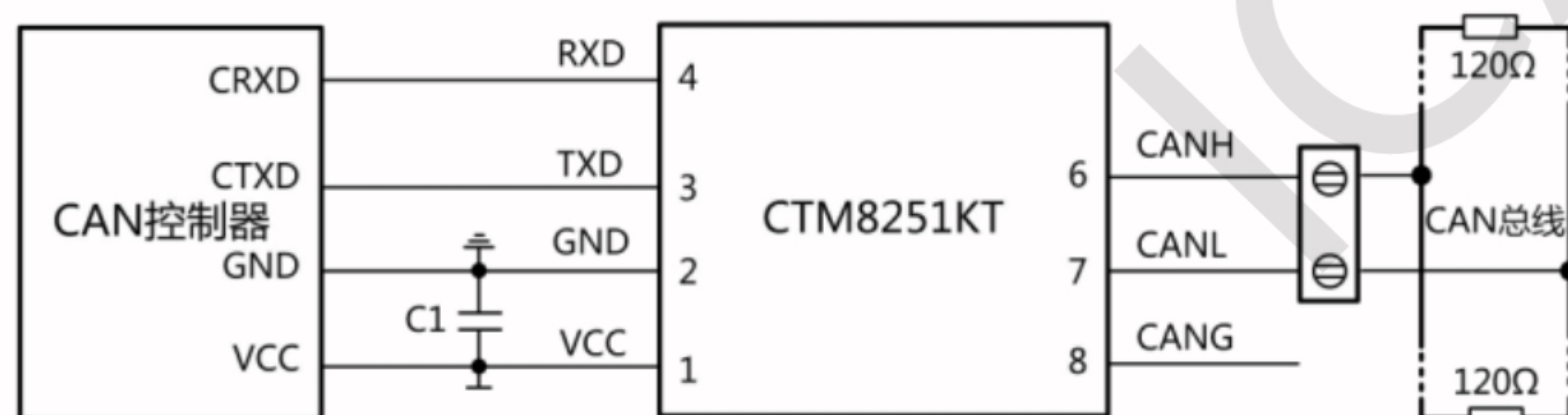
图 1.CAN控制器 5V供电应用电路
