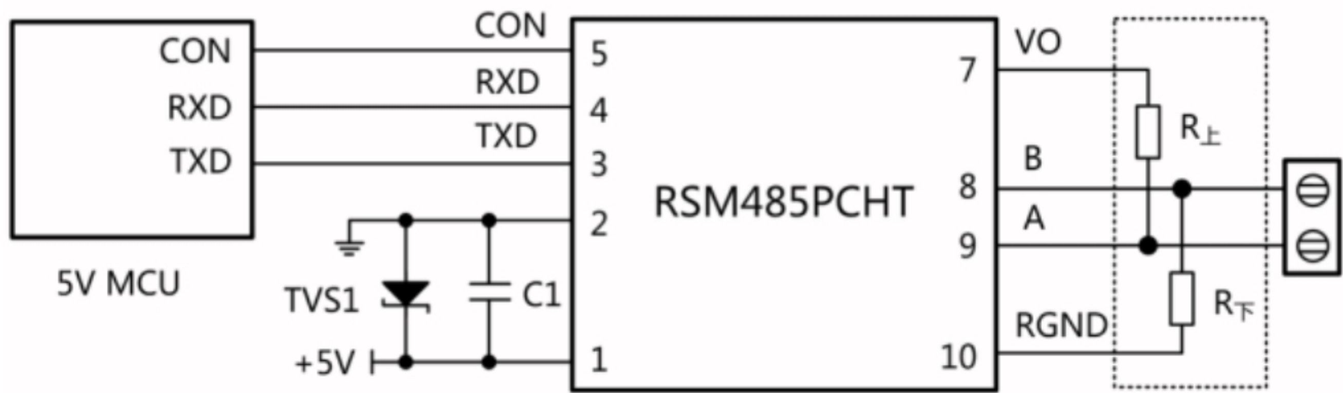
图3.MCU 5V供电应用电路
