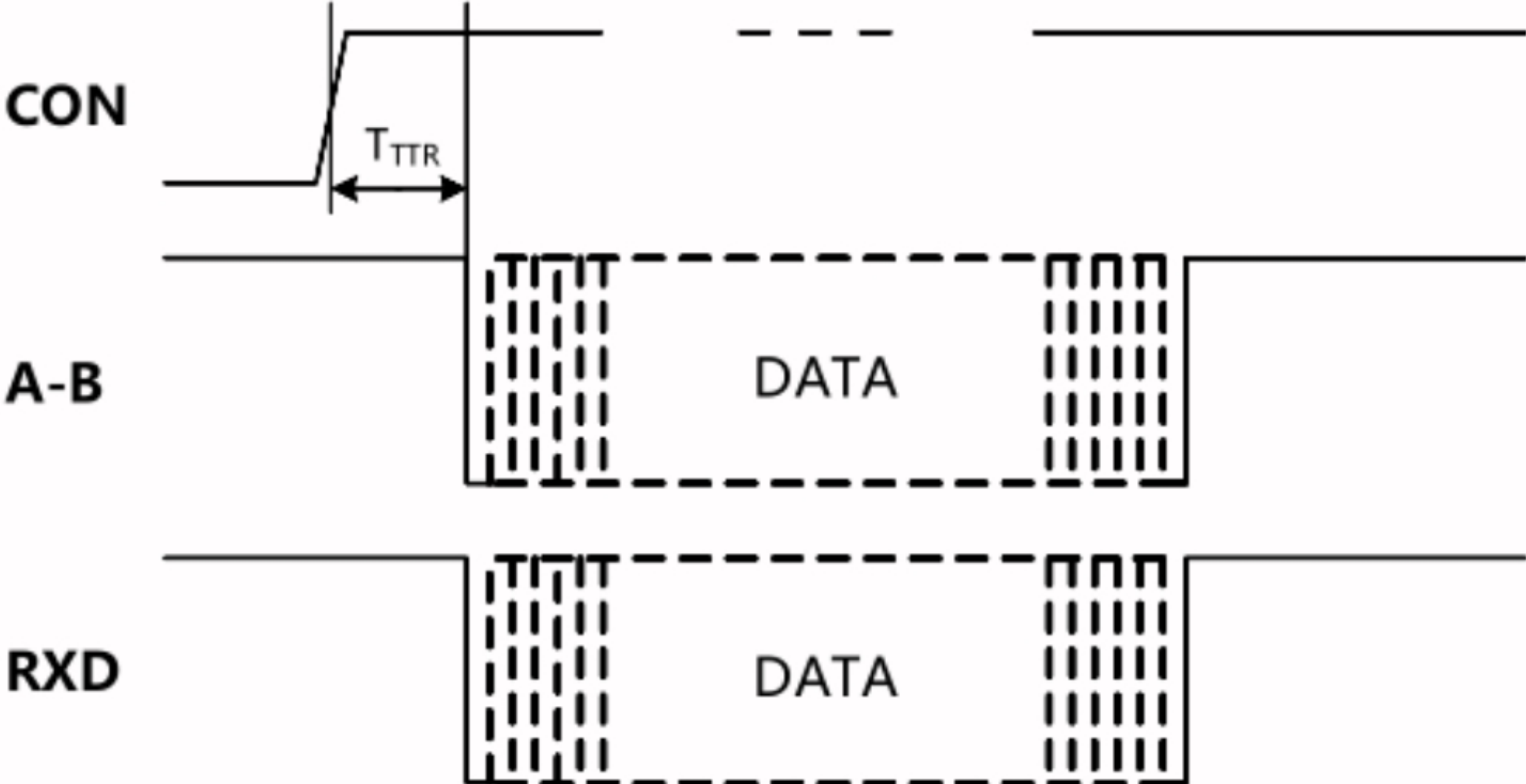
图2. RSM(3)485PCHT模块数据接收时序图
