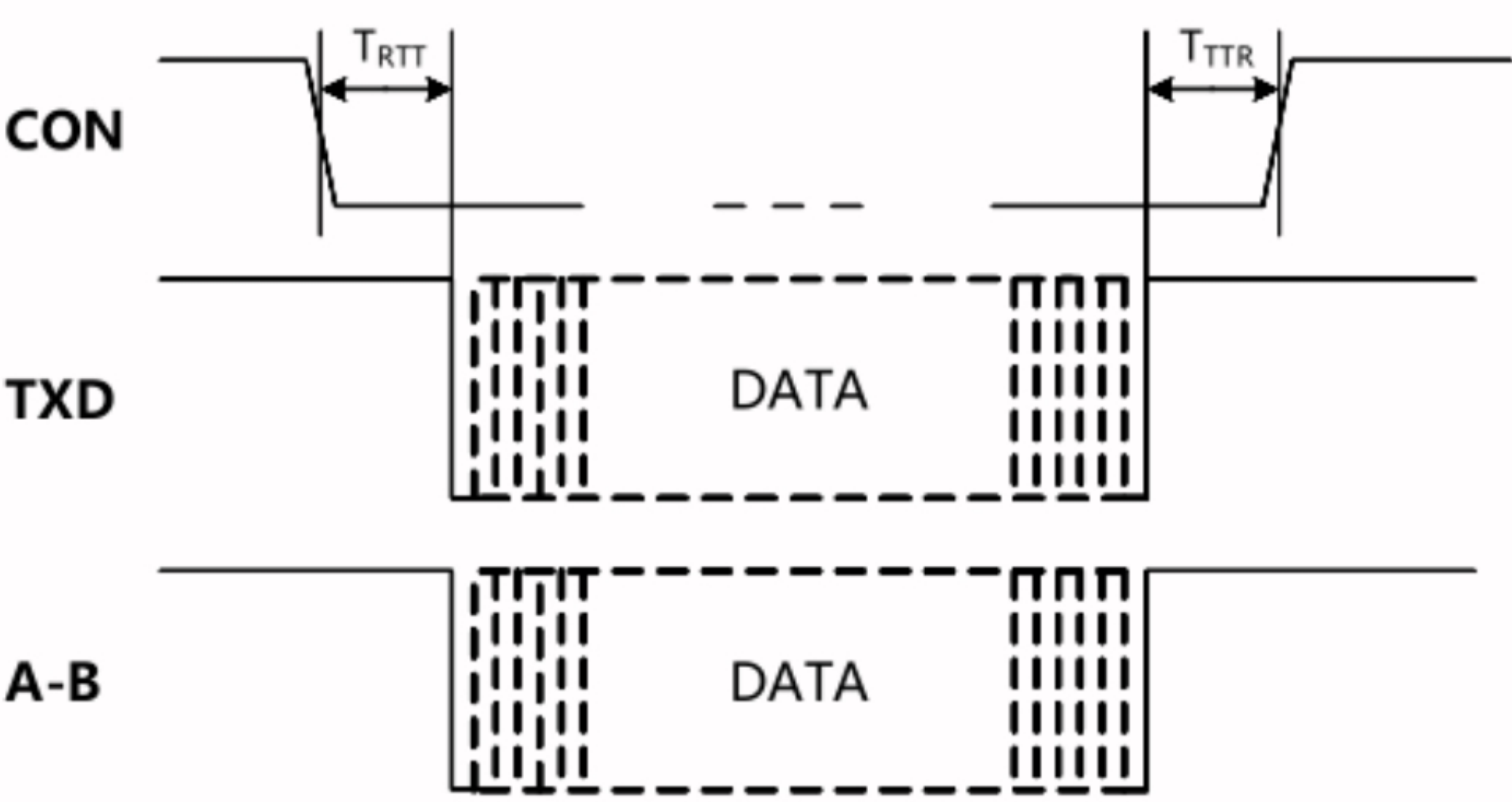
图1. RSM(3)485PCHT模块数据发送时序图
