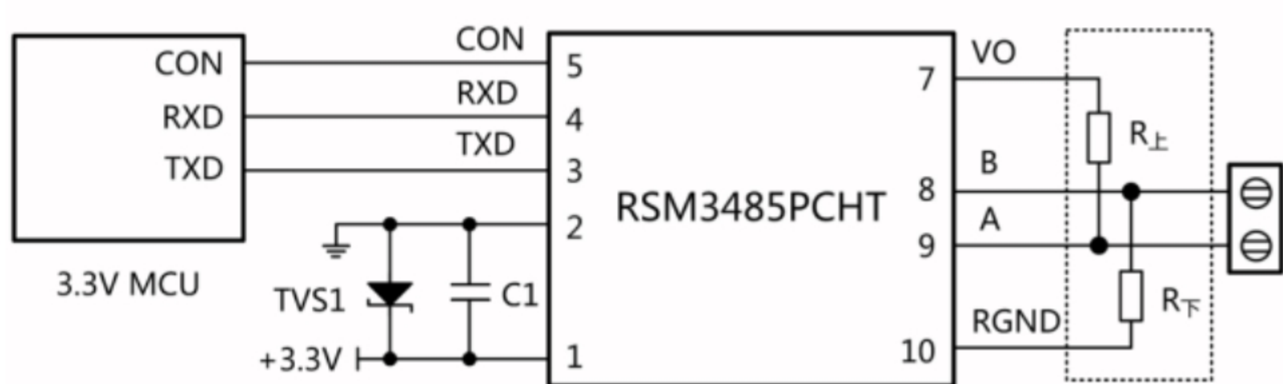
图4.MCU 3.3V供电应用电路
