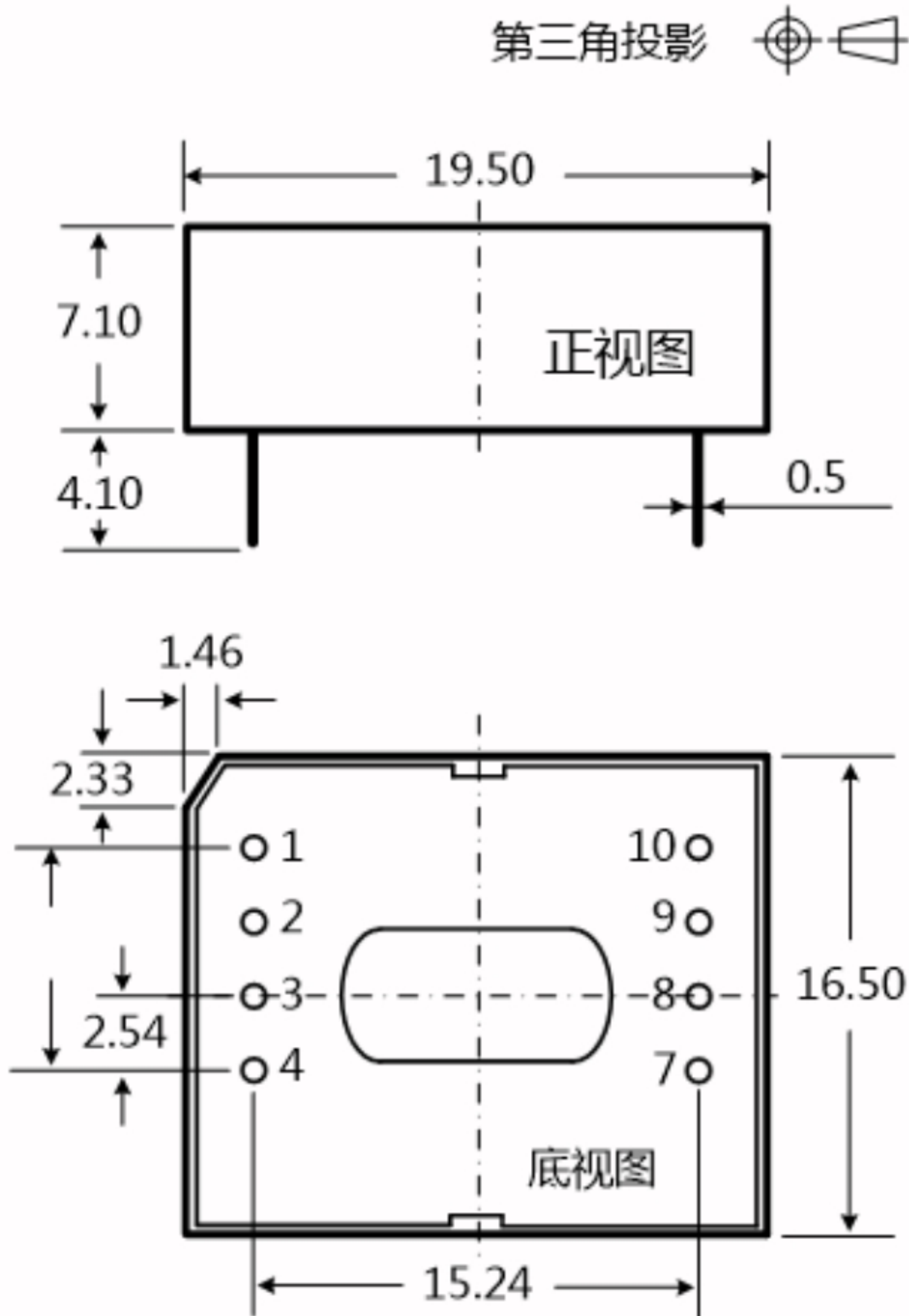
外观尺寸图
