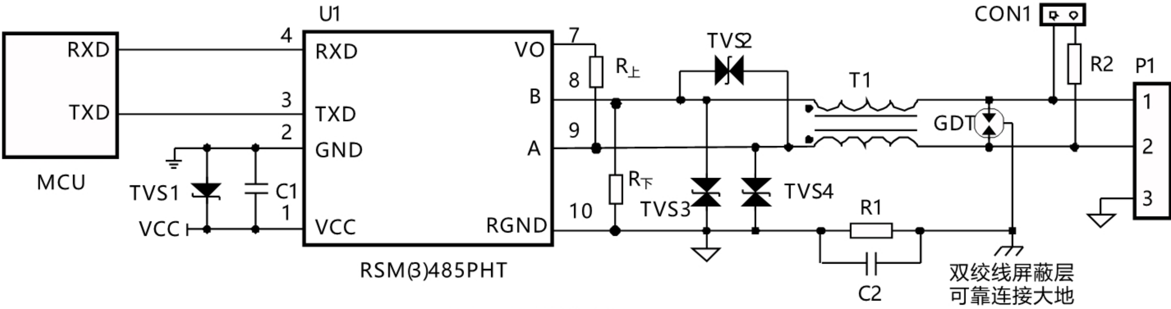
图3. EMC推荐电路
