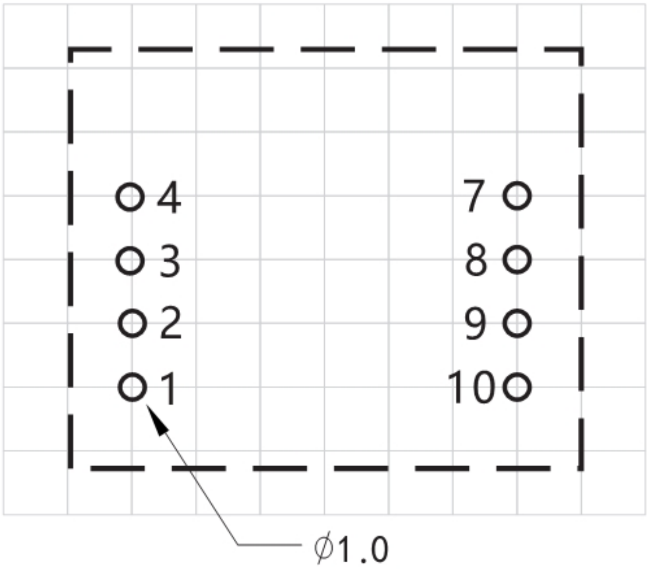
引脚定义
