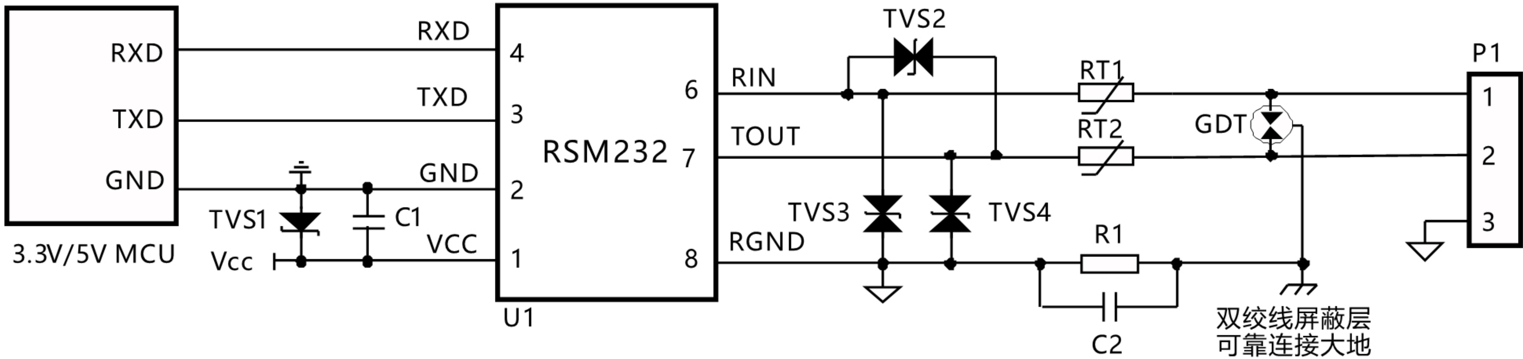
图3. EMC推荐电路
