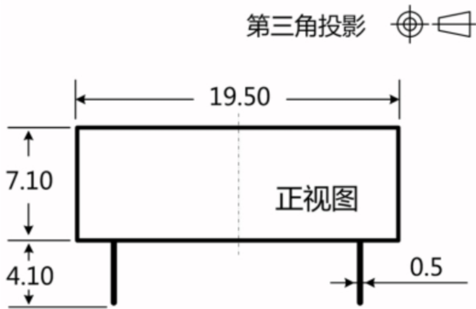
外观尺寸图
