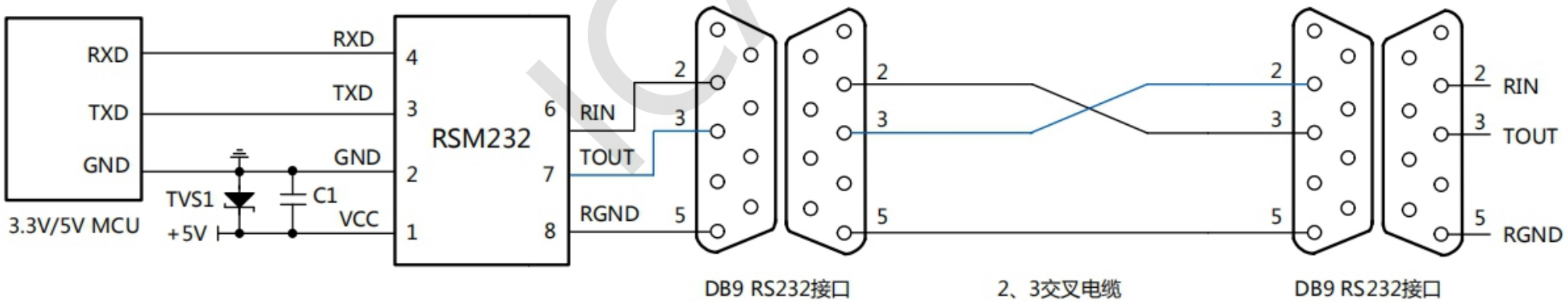
图 2. 使用 2、3 脚交叉串口线
