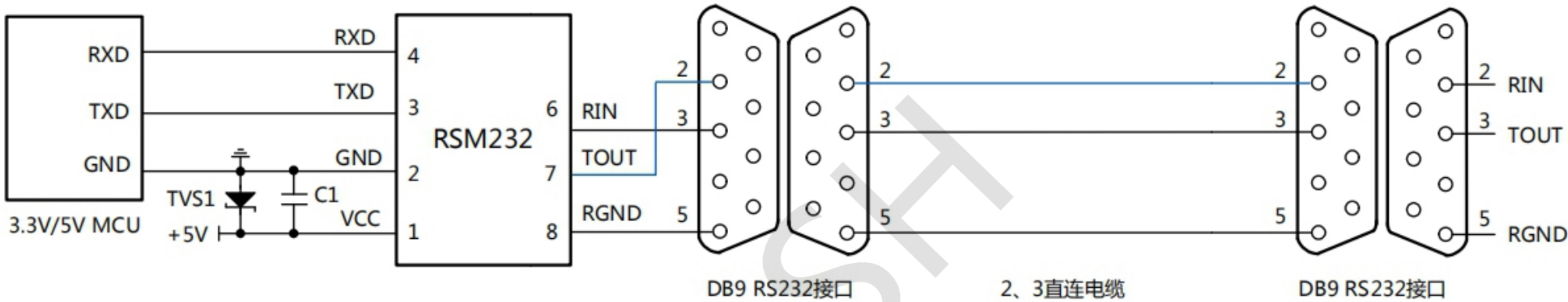
图1. 使用 2、3 脚直连串口线
