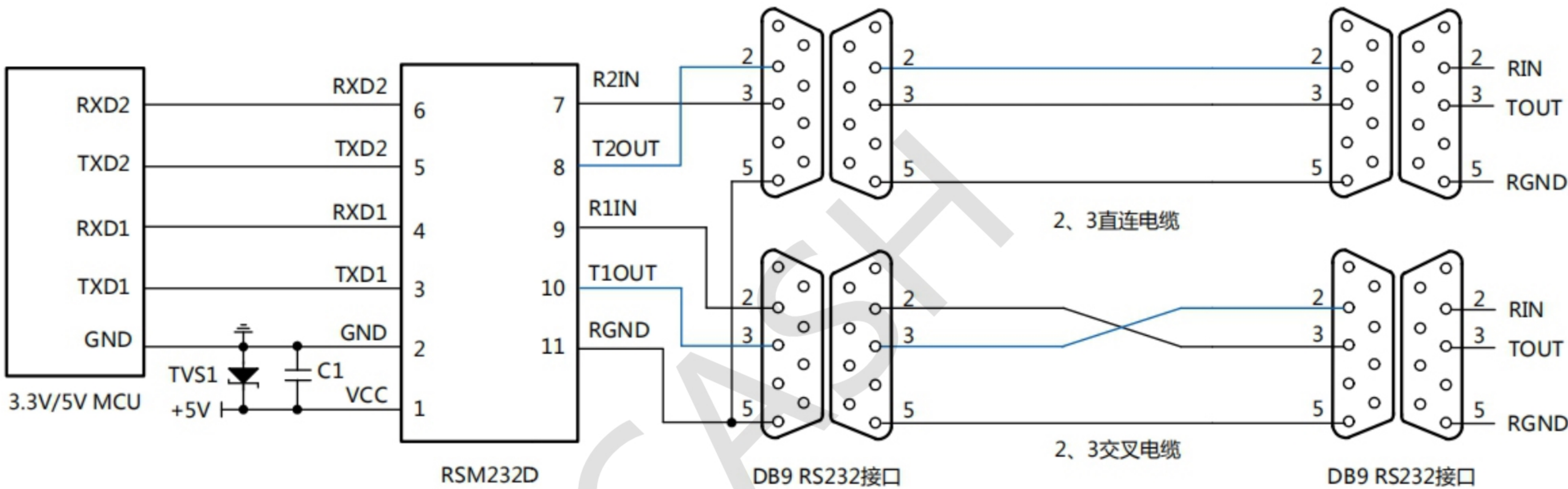
图1. 典型连接电路图
