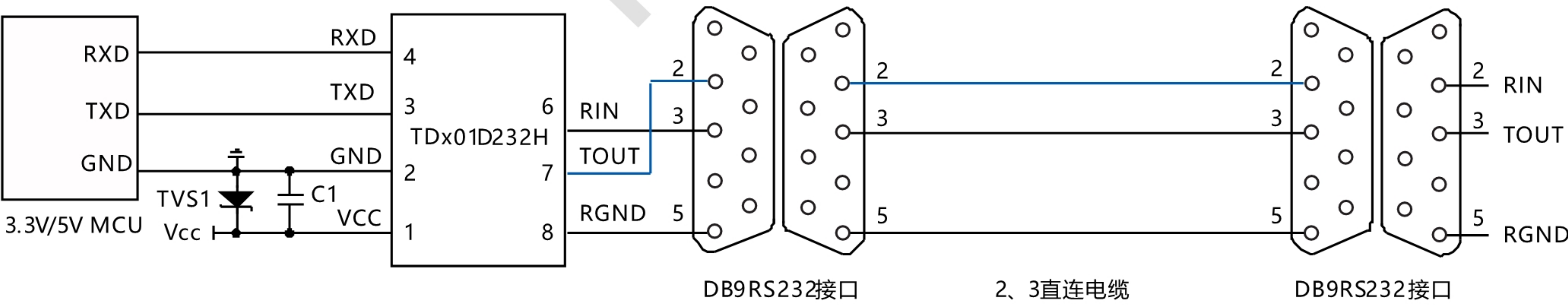
图1. 使用 2、3 脚直连串口线
