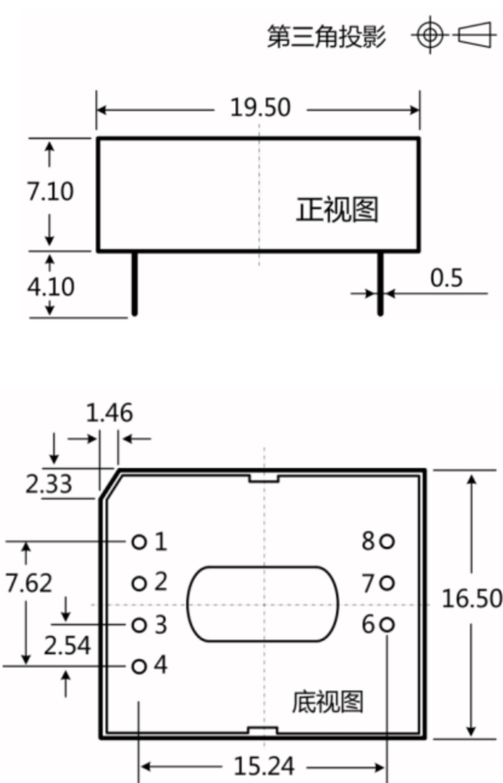
外观尺寸图
