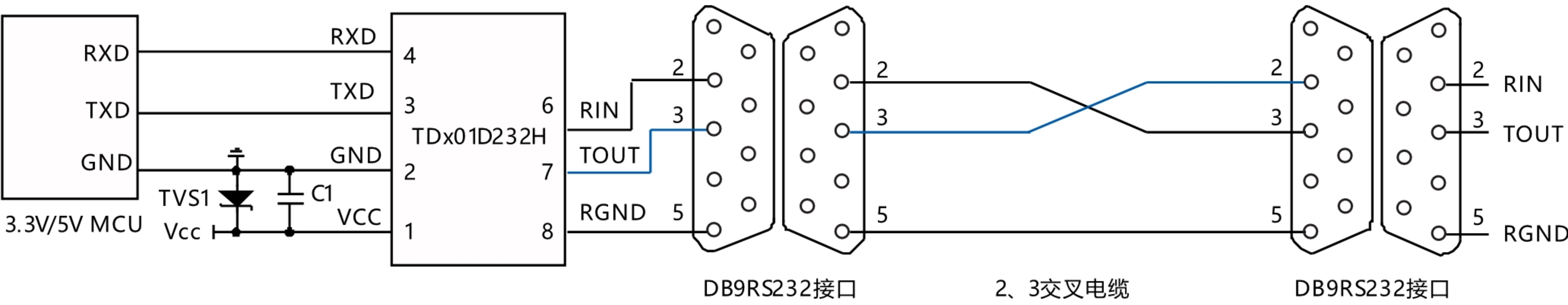
图 2. 使用 2、3 脚交叉串口线
