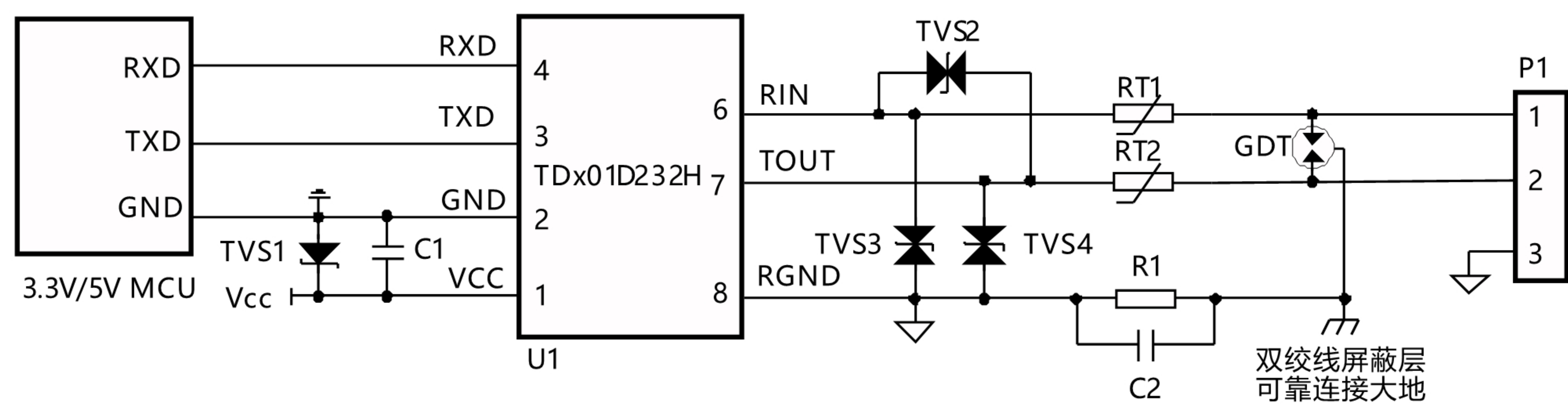
图3. EMC推荐电路
