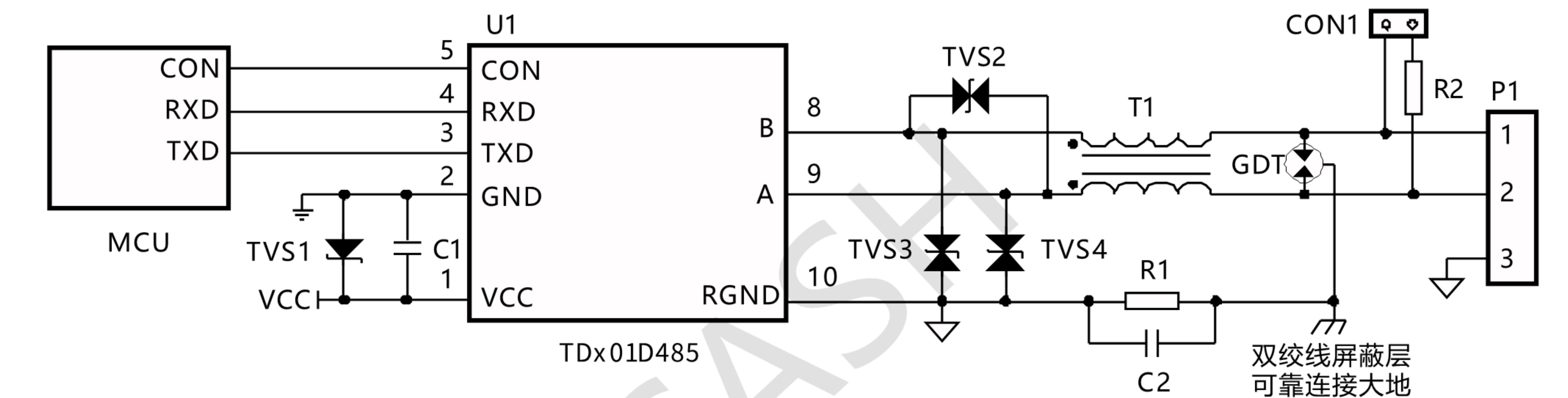
图5. EMC推荐电路
