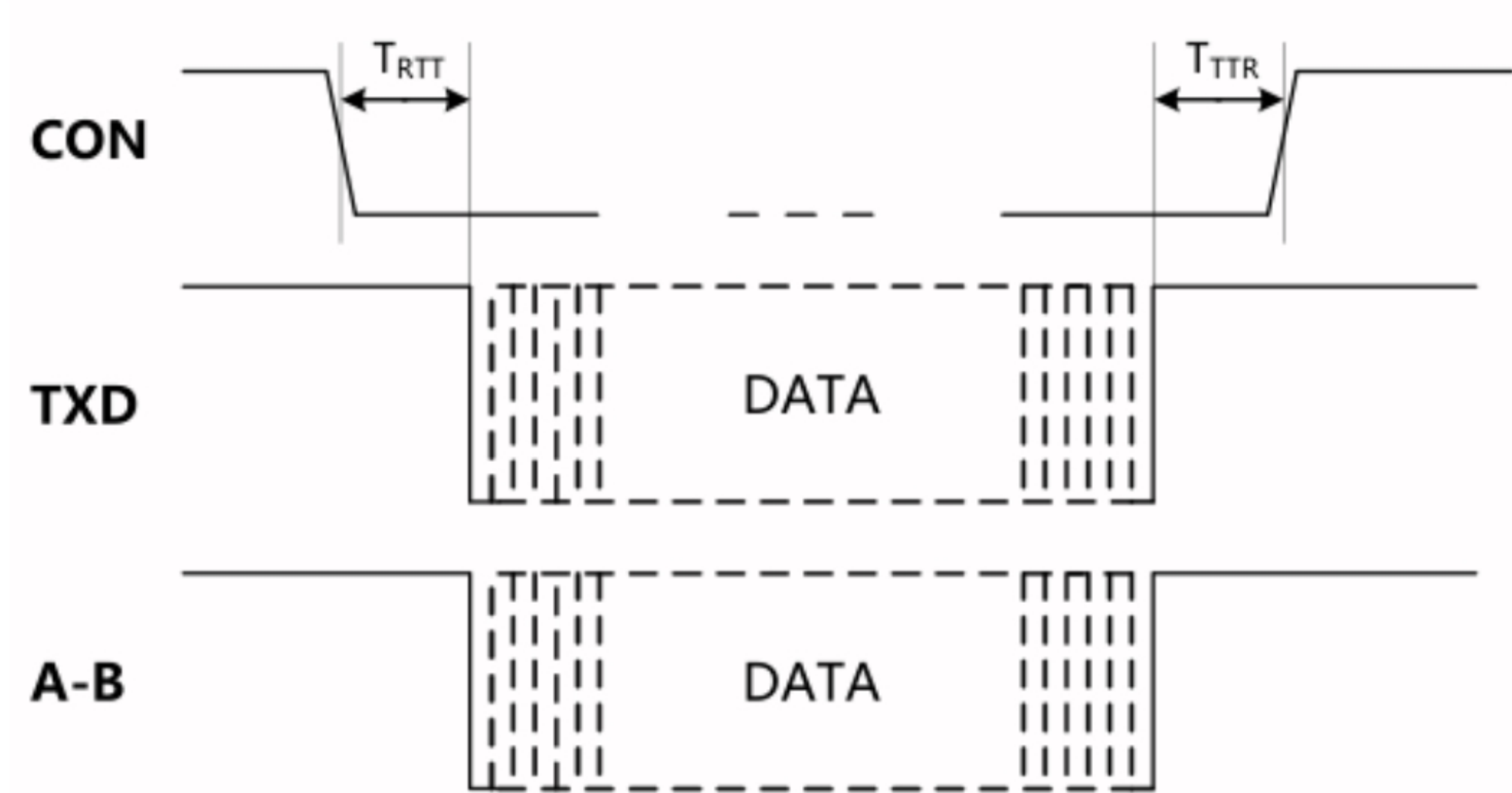
图1. TDx01D485模块数据发送时序图
