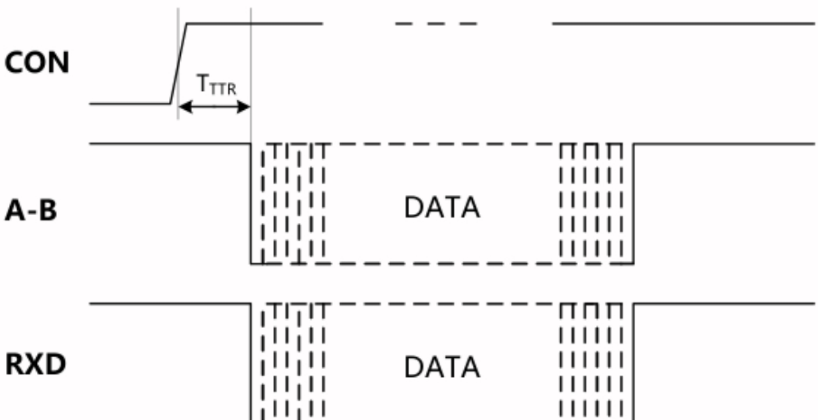
图2. TDx01D485模块数据接收时序图
